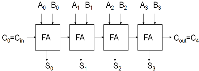
Fig.8.4:4-bRippleCarryAdder.
