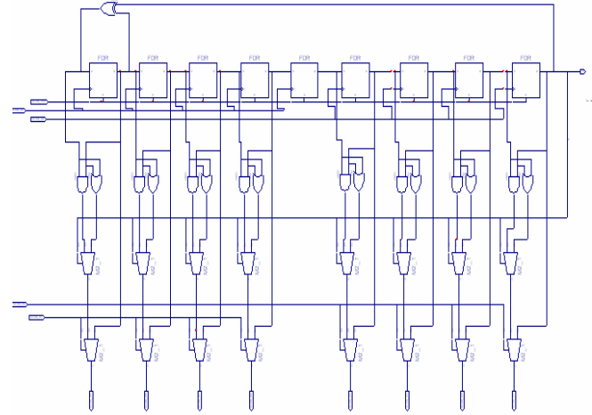
Fig.5. LP-LFSR.
