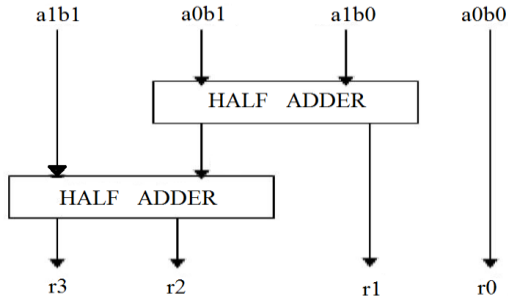
Fig.4. Block diagram 2x2 Vedic multiplier.
